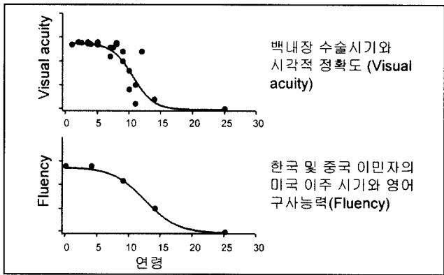
Fig. 1. 사람에게서 보이는 Critical period의 대표적 예. 전 생애 중 어렸을 때의 경험이 대뇌피질의 발달을 가져와서 그 경험이 관여하는 행동수행능력을 최대한 시키는 예를 볼 수 있다.
