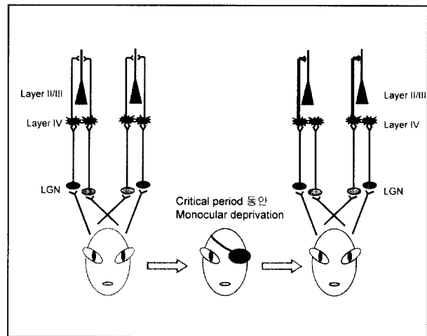
Fig. 3. Critical period. 눈으로 들어온 빛은 망막에서 신경세포를 타고 lateral geniculate nucleus (LGN)을 거쳐서 시각피질의 layer IV 세포로 전달 된다. Layer IV 세포는 양쪽 눈의 신호를 모두 받는 layer II/III 세포와 신호를 주고 받으면서 전달된 시각 정보를 저장, 제어, 가공하게 된다. 이때 만약 생후 초기의 특정 기간 동안 한쪽 눈을 가림으로써 (monocular deprivation) 시각신호의 입력을 차단하면 해당하는 눈으로부터 들어오는 layer IV 세포와 layer II/III 세포의 시냅스가 퇴출되게 되어 이후 평생토록 해당 눈으로부터의 신호를 받지 못하게 된다. 이러한 생후 초기의 특정 기간을 critical period 라고 한다.
