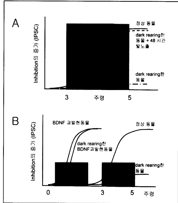
Fig. 4. Dark rearing 효과와 inhibition의 발달. (A) 생쥐 시각피질에서의 inhibitory neuron의 활성을 측정하면 생후 3주-5주의 기간동안 활성이 증가함을 볼 수 있다. 만약 생쥐를 태어나서부터 어두운 방에서 키워 시각경험을 차단하면 (dark rearing) 이시기의 inhibition의 증가양상이 사라진다. 그런데 5주가 되기 전 약 2일 동안 빛에 노출시키면 거의 정상상태의 inhibition을 확보하는 것을 알 수 있다. 이는 critical period 동안의 시각경험이 (단 2일 정도라도) inhibition을 발달시키는데 중요한 역할을 함을 암시한다. (B) BDNF가 과발현된 형질전환동물은 inhibition의 발달이 생후 직후부터 일어나기 시작하여 일찍 완료된다. 또한 이들은 dark rearing 시에도 정상적인 inhibition의 발달을 가져온다. 따라서 경험과 inhibition의 발달 가운데에서 BDNF가 중요한 역할을 함을 알 수 있다.
