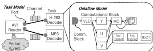
그림 2 알고리즘 명세의 예 (DivX 동영상 플레이어)
