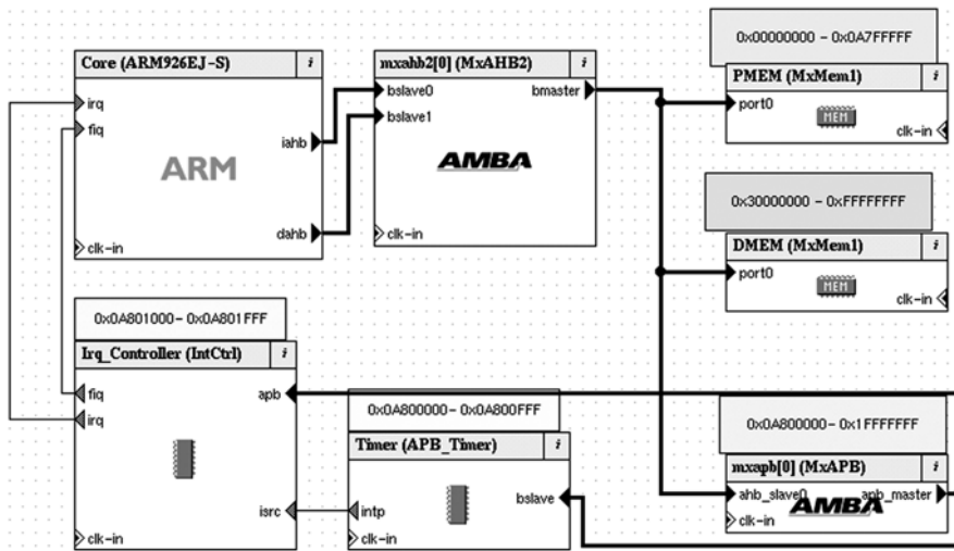
그림 10 SoC Designer를 이용한 실험 플랫폼 명세
