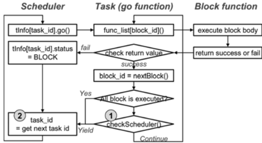
그림 7 생성된 코드의 동작 구조
