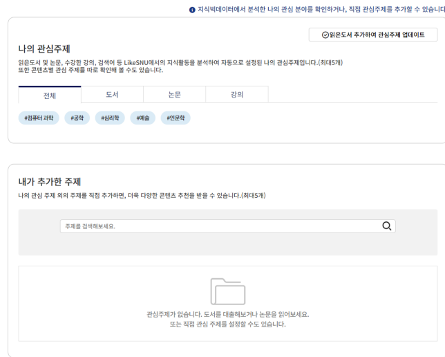
그림 21 관심주제 설정
