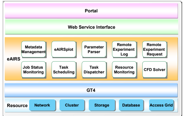
그림 2. e-AIRS 구조
