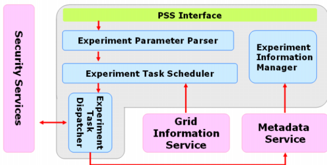
그림 1. PSS 구조
