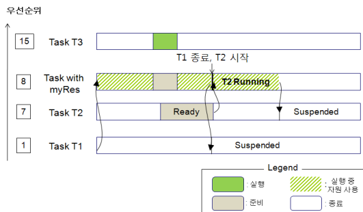
Fig. 4 내부 자원 사용에 따른 우선순위의 변화
