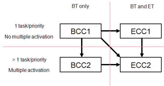
Fig. 7 Conformance Class의 분류
