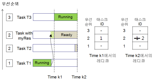
Fig. 12 우선순위 변경으로 인한 CCI 레디큐 문제
