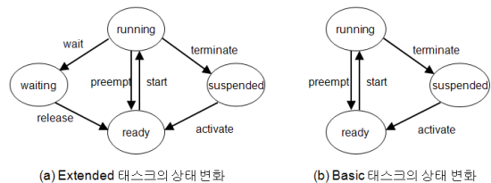
Fig. 1 태스크의 상태 변화
