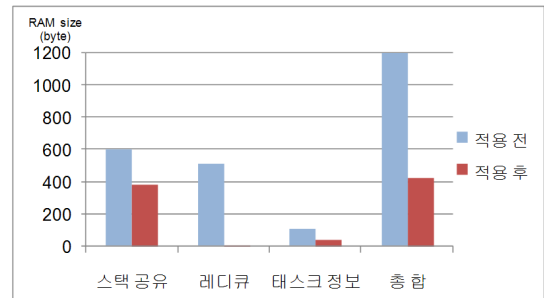
Fig. 23 정량적인 메모리 절약 분석
