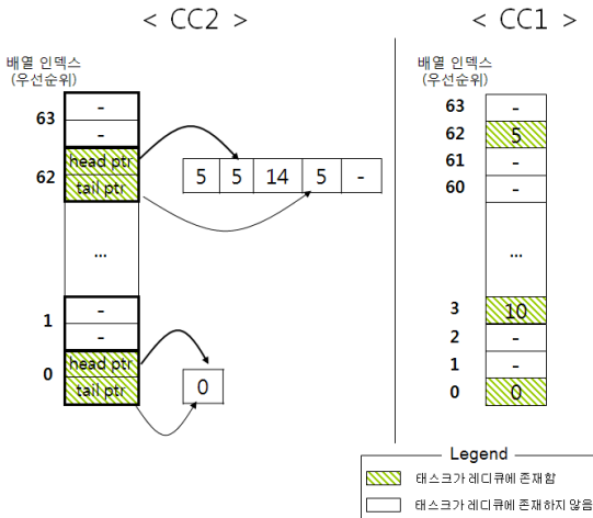
Fig. 10 CC1과 CC2의 레디큐 구현
