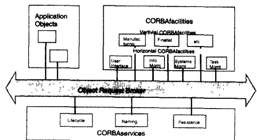
<그림 1> OMA(Object Management Architecture) [출처 OMG]
